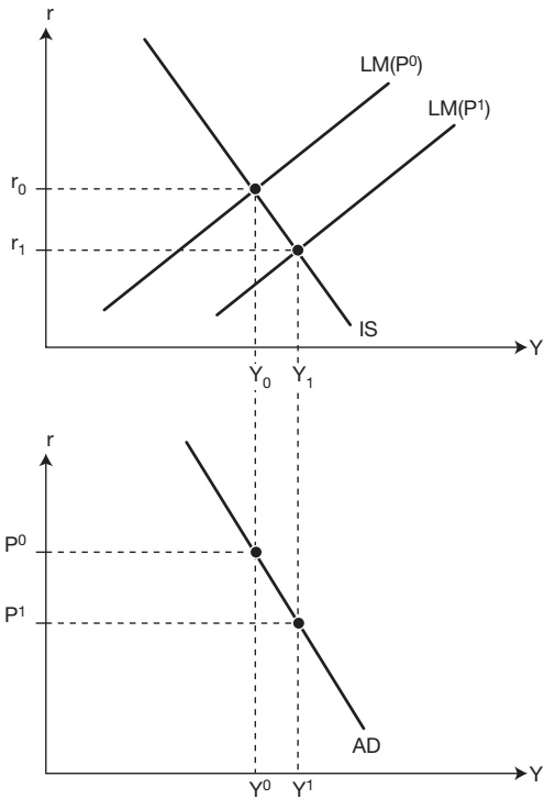
Figur 8a.: Udedning af AD-kurven ud fra IS-LM-modellen
