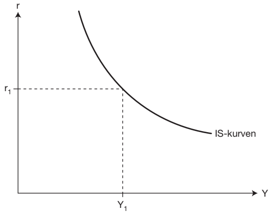
Figur 3. IS-kurven
